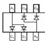
BAT54AD
