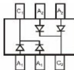
BAT54CD
