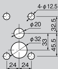
パネル穴明け寸法 Panel drilling dimensions
