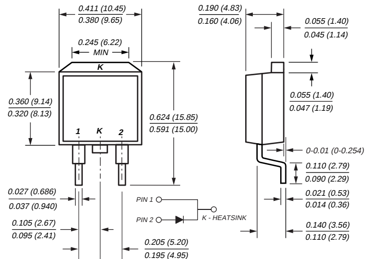
TO-263AB (SBLB10L25)
