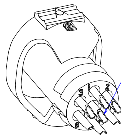
VIEW Y
