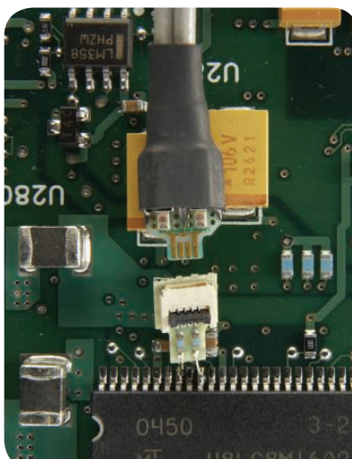
InfiniiMax ZIF tip soldered on board
