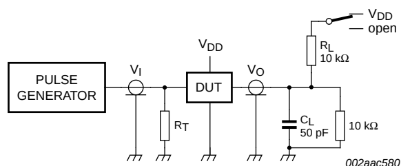
Fig 16. Test circuitry for enable/disable times, SDOUT ( t_{en}(SDOUT) and t_{dis}(SDOUT) )
