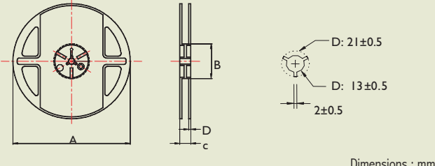
Reel Dimensions
