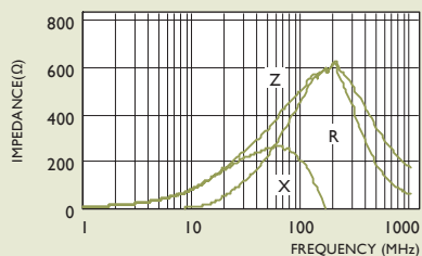
PBY160808T-501Y-S
