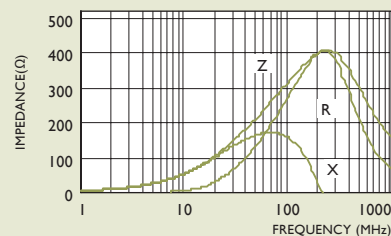
PBY160808T-301Y-S
