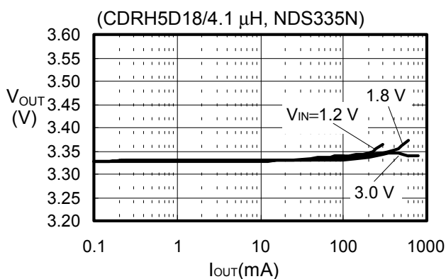
(7) S-8341A33AFT
