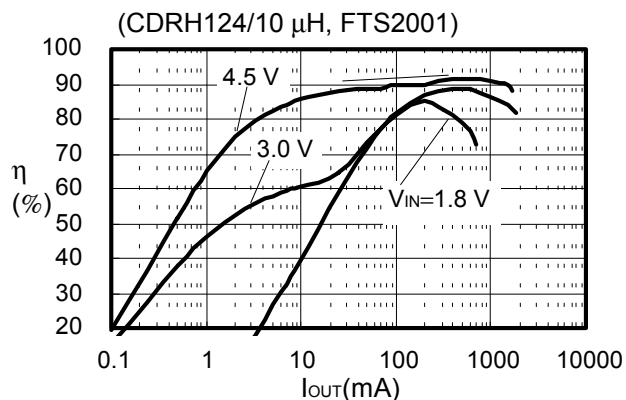
(14) S-8340C25AFT
