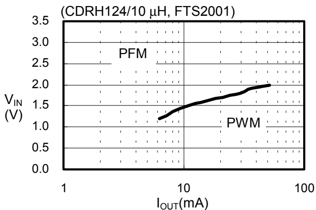
(32) S-8341C25AFT
