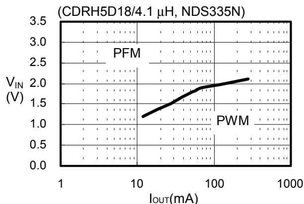
(27) S-8341A33AFT
