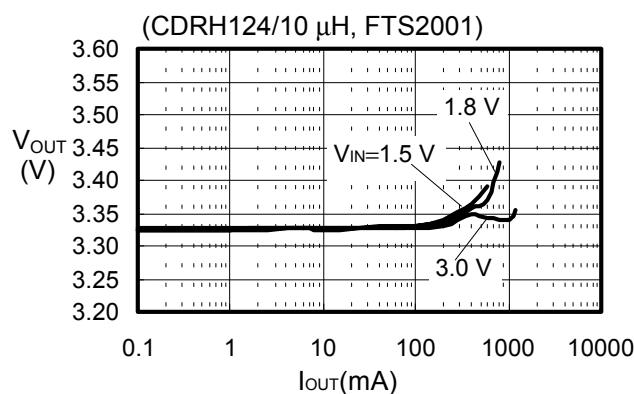
(8) S-8341A33AFT
