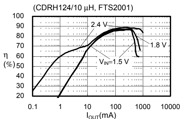
(16) S-8341C25AFT
