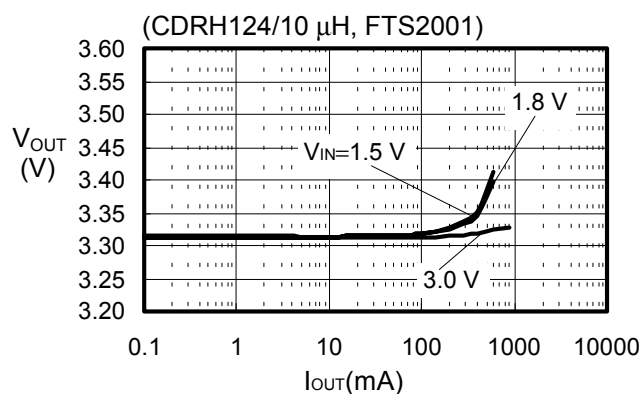
(8) S-8341A33AFT
