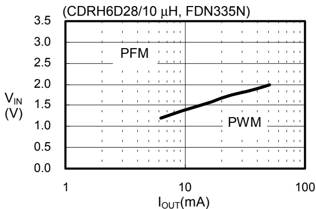
(31) S-8341C25AFT
