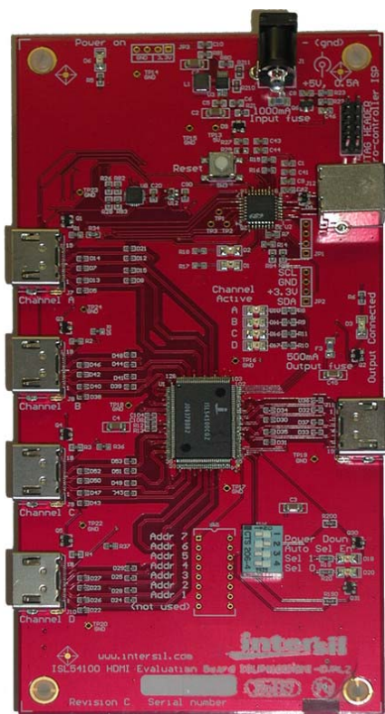
ISL54100A (4→1) ISL54100AHDMI-EVALZ
