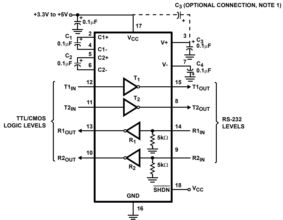
ISL83385E (Note 2)
