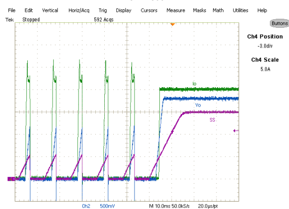
Fig. 26: Short (Hiccup) Recovery Ch 2 : V_{out} , Ch 3 : V_{SS} , Ch 4 : I_o
