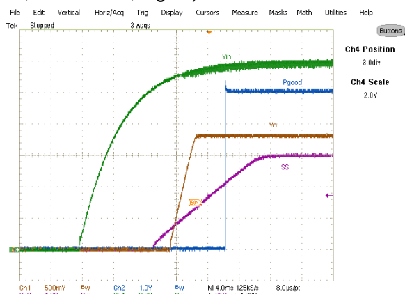
Fig. 22: Start up at 25A Load Ch 1 : V_o , Ch 2 :PGood Ch 3 : V_{SS} Ch 4 : V_{in}
