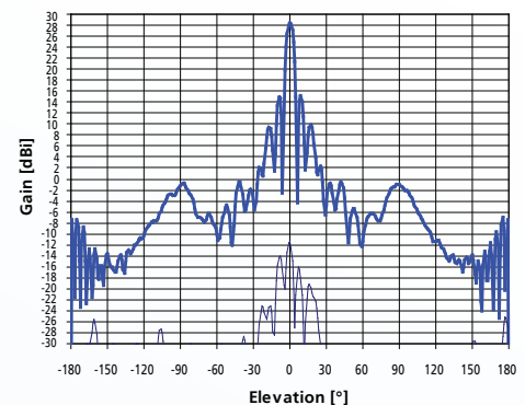
5.7GHz E-Plane
