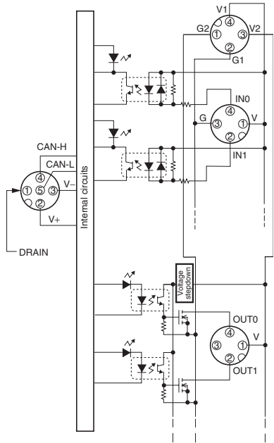
DRT2-MD16CL (NPN)
