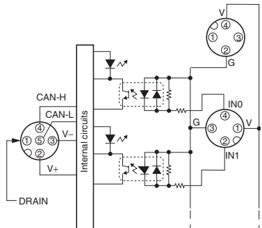
DRT2-WD16CL-1 (PNP)
