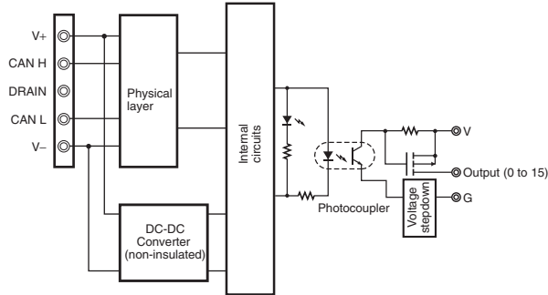
DRT2-OD16ML(X)-1
