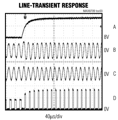
A: V_{BATT} , 5V/div B: V_{IFB} , 2V/div C: V_{VFB} , 2V/div D: V_{LX1} , 10V/div
