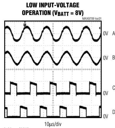
A: V_{IFB} , 2V/div B: V_{VFB} , 2V/div C: V_{LX1} , 10V/div D: V_{LX2} , 10V/div
