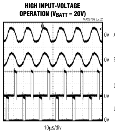
A: V_{IFB} , 2V/div B: V_{VFB} , 2V/div C: V_{LX1} , 10V/div D: V_{LX2} , 10V/div
