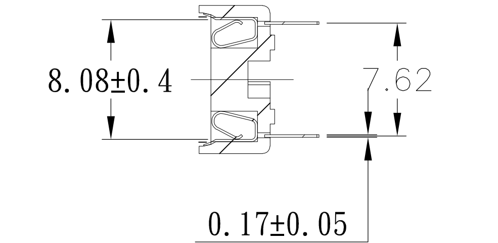
SECTION D-D
