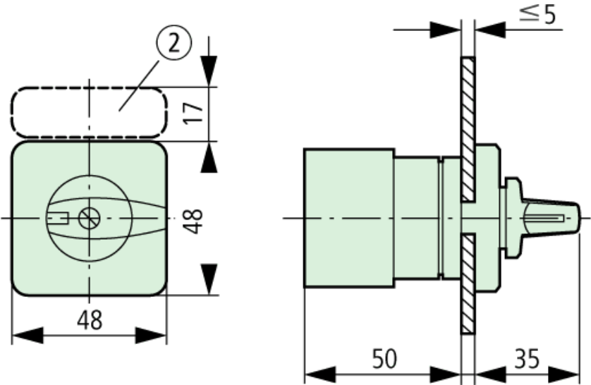
Dimensions
