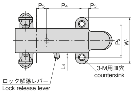
C-1157-1-A (平行取付けタイプ) (Parallel installation type)
