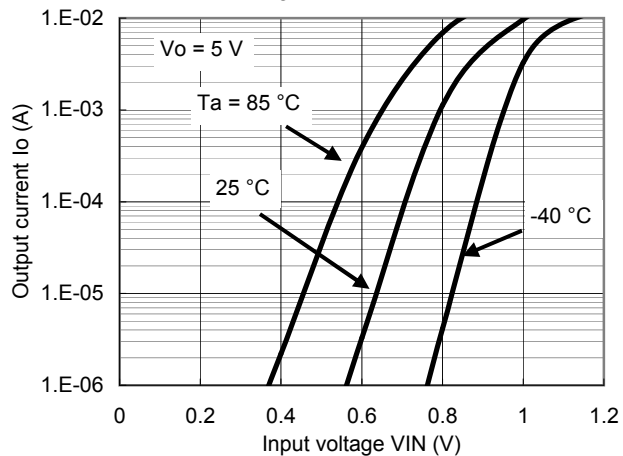
Io - VIN
