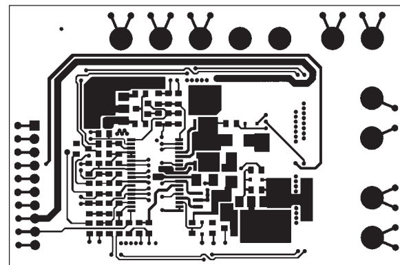
Copper Layer 4
