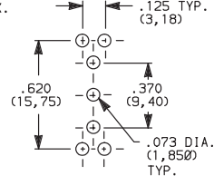
E112SD1_BE SPDT
