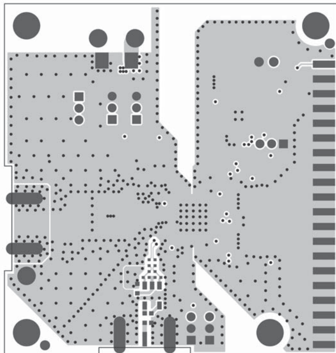
Bottom Side
