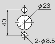
パネル穴明け寸法 Panel drilling dimensions
