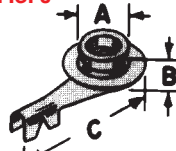
Stud w/Crimp Lugon
