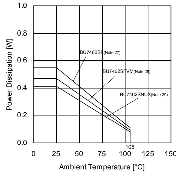
(f) BU7462Sxxx
