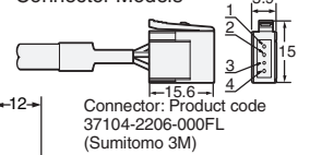
Diagram 15 E2E-X14MD□/E2E-X10ME□/F□ E2E-X10MY□
