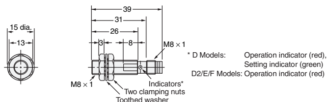
Diagram 28 E2E-X2D□-M3G/E2E-X1R5E□-M3/X1RF□-M3
