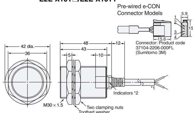
Diagram 16 E2E-X10D□/E2E-X10E□/F□ E2E-X10Y□/E2E-X10T1
