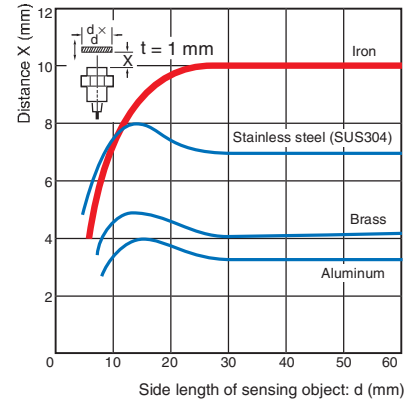
E2E-X10ME/-X10MY/-X10MF
