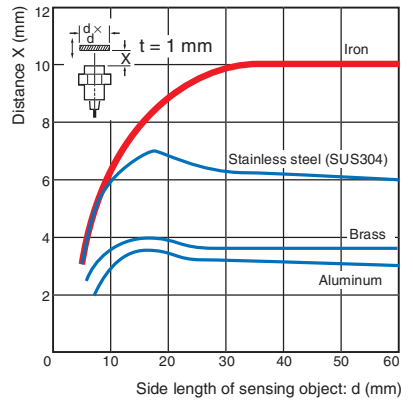
E2E-CR8
