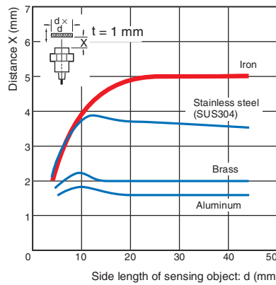
E2E-CR6
