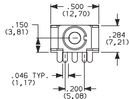
8121SD9RGE SPDT
