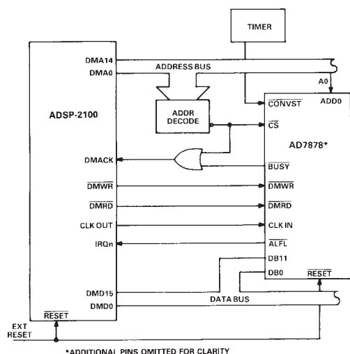
Figure 18. AD7878-ADSP-2700 Interface
