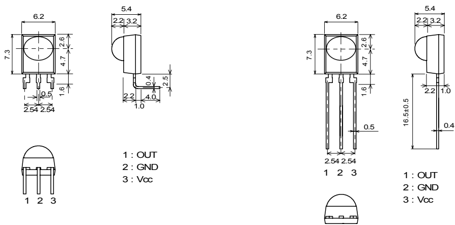
NJL21H000A UNIT:mm
