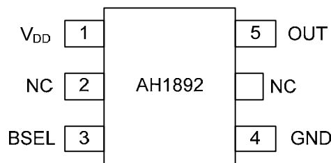
SOT553
