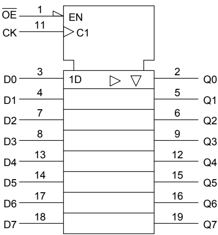
論理図
