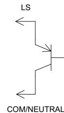
PNP O.C. TRANSISTOR OR (P) FET INPUT
