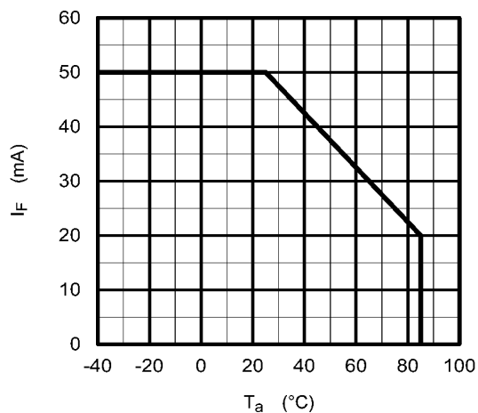
図 12.1.1 I_F - T_a
