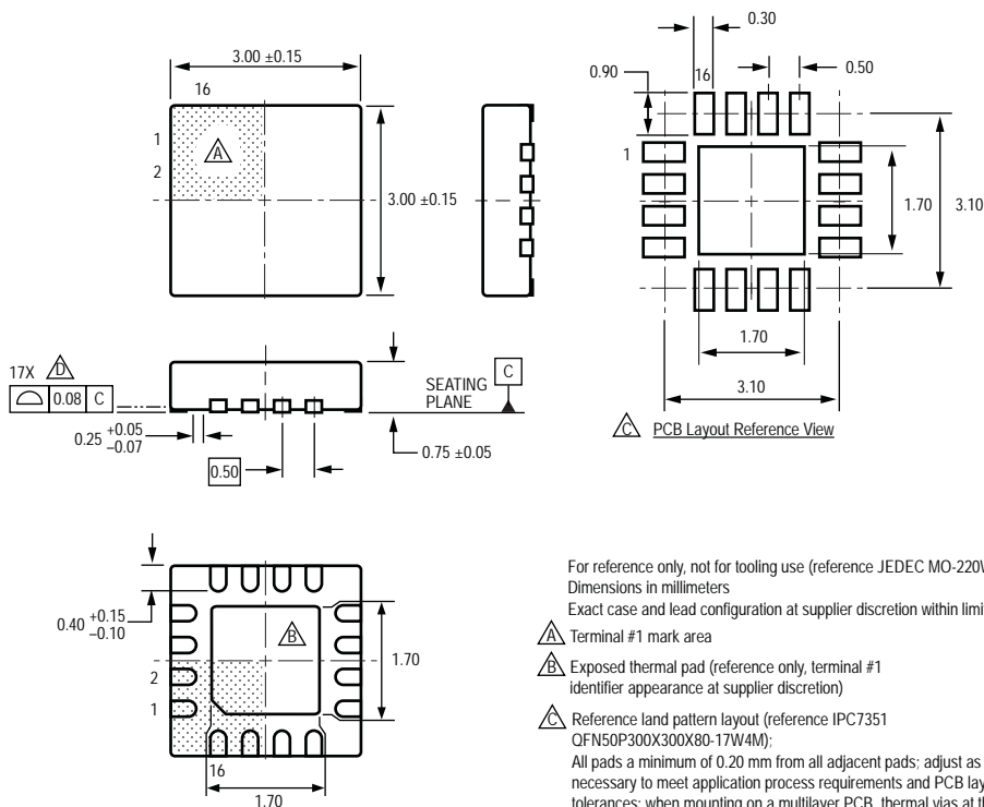
ES Package, 16-Contact QFN
