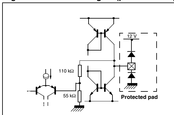
Figure 16. I²C bus (SDA) (pin 56)
