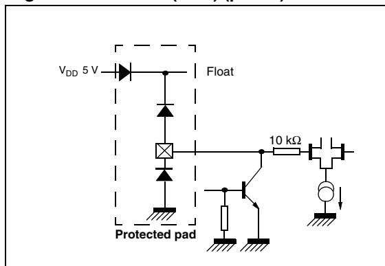
Figure 16. I²C bus (SDA) (pin 56)
