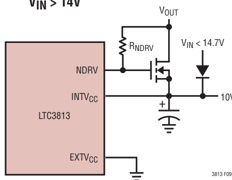
(d) INTV CC from V_{OUT} , V_{OUT} > 15V
