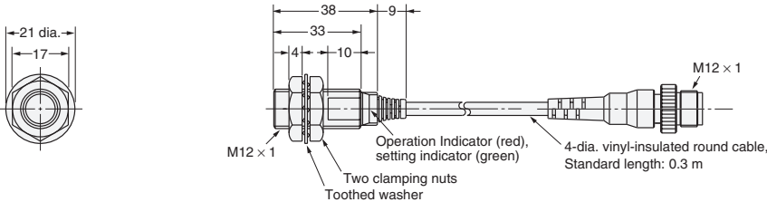
Fig. 30: E2E-X3D1-M1GJ E2E-X3D1-M1J-T
