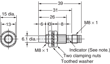
Fig. 29: E2E-X4MD□-M3G/E2E-X2ME□-M3/F□-M3
