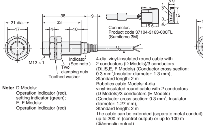
Fig. 9: E2E-X3D-N E2E-X2E/F
