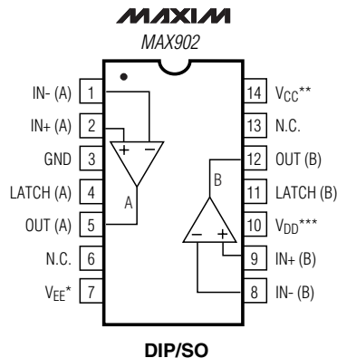
DIP/SO
