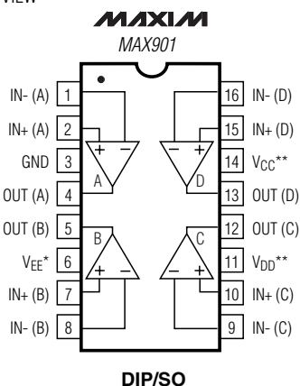
DIP/SO
