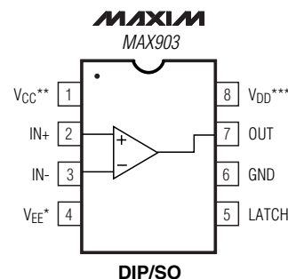
DIP/SO
