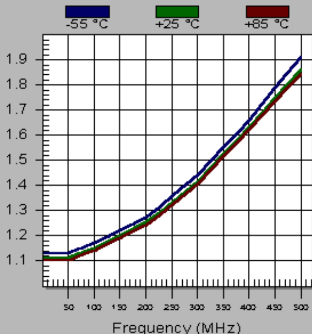
TM6505 Output VSWR
