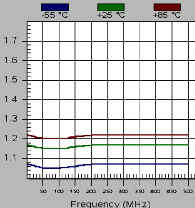
TM6505 Input VSWR
