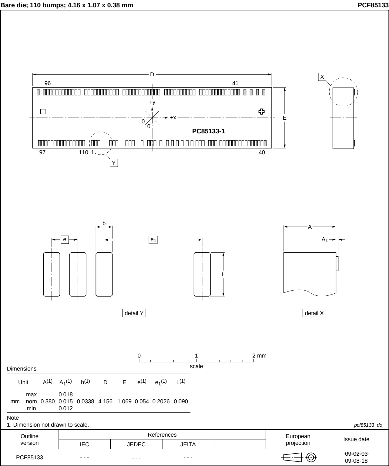
Fig 24. Bare die outline of PCF85133
