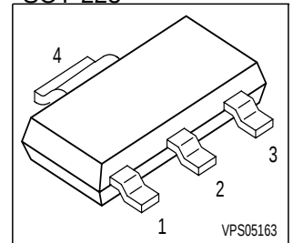
SOT-223
