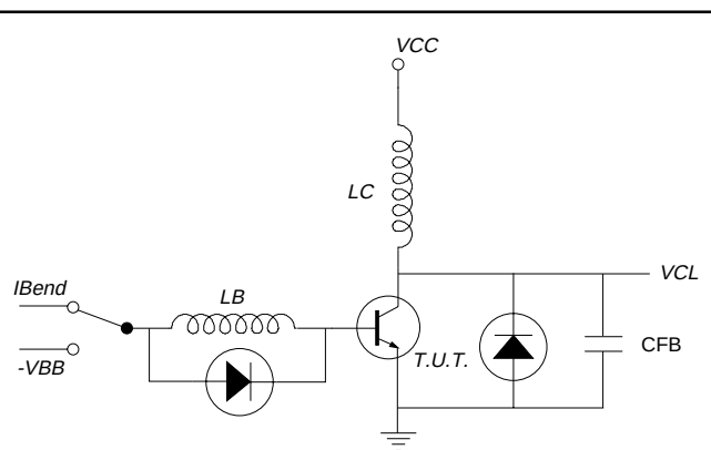
Fig.15. Test Circuit RBSOA.
