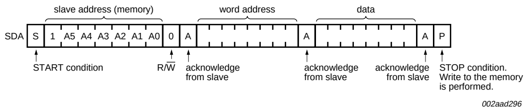
Fig 12. Byte write
