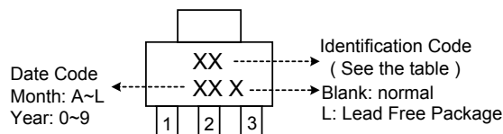
(4) SOT89-3L
