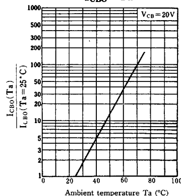
I_{CBO} - T_a
