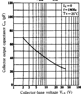
C_{ob} - V_{CB}
