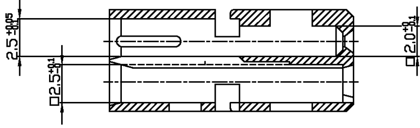
SECT B-B (SCALE: 4-1)
