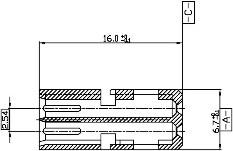
SECT A-A (SCALE: 4-1)
