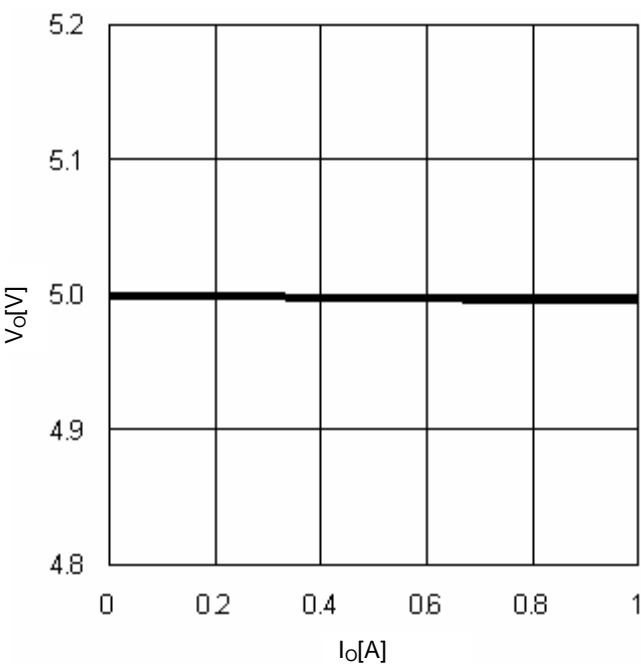
Fig.12 I_O - V_O
