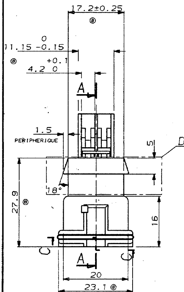
DETAIL D: PARTIE SUPERIEURE PORTE-MODULE
