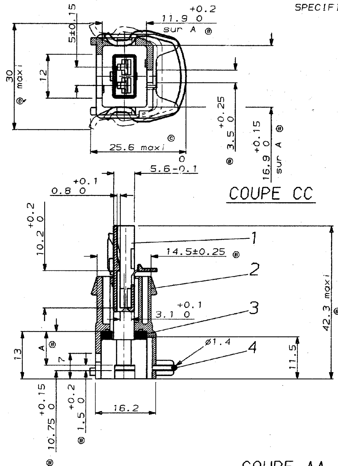
COUPE AA
