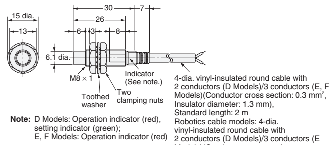
Fig. 6: E2E-X4MD□ E2E-X2ME□/F□
