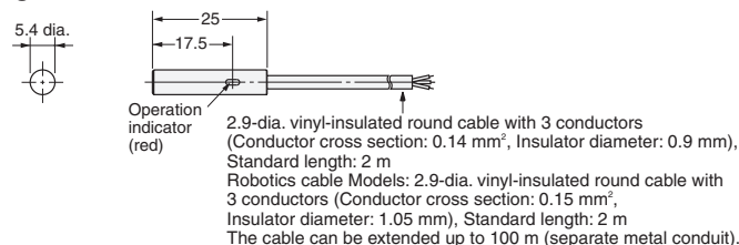
Fig. 4: E2E-X1□□
