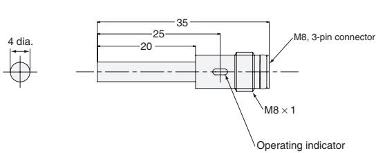
Fig. 36: E2E-CR8□□-M5
