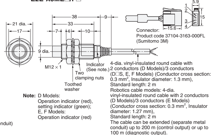
Fig. 10: E2E-X8MD□ E2E-X5ME□/F□
