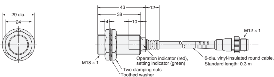
Fig. 32: E2E-X7D1-M1GJ E2E-X7D1-M1J-T
