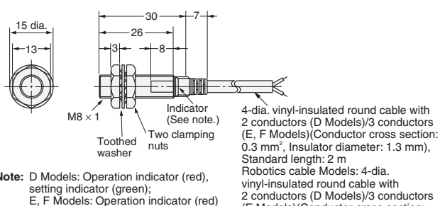
Fig. 5: E2E-X2D□-N E2E-X1R5E□/F□
