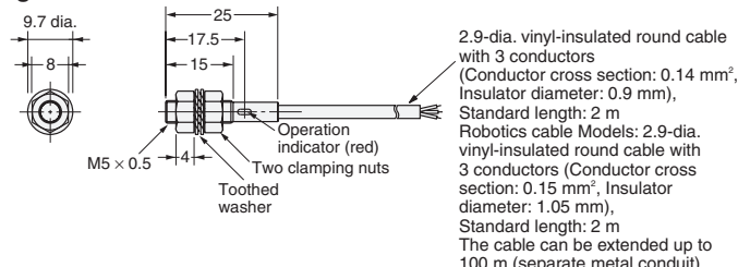
Fig. 4: E2E-X1□□
