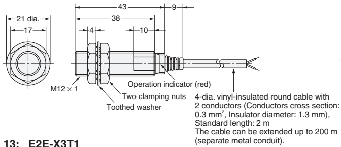
Fig. 13: E2E-X3T1
