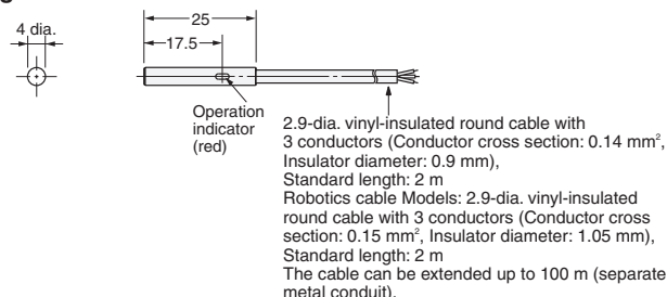
Fig. 2: E2E-CR8□□
