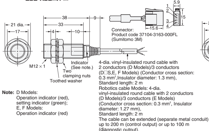
Fig. 9: E2E-X3D□-N E2E-X2E□/F□
