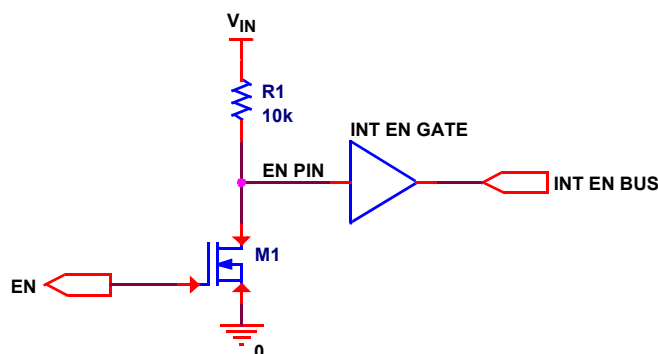
FIGURE 28. ENABLE
