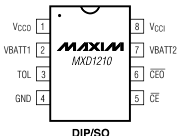
DIP/SO
